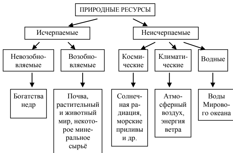
Рис. 13. Классификация природных ресурсов по степени истощаемости
