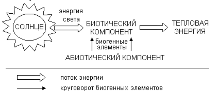
Рис. 3. Поток энергии и круговороты биоогенных элементов в экосистеме
