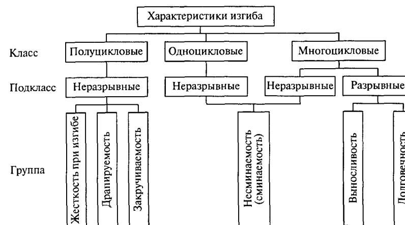
Рис. 4.25. Классификация характеристик изгиба материалов
