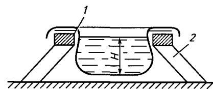
Рис. 4.43. Определение водоупорности методом «кошеля»
