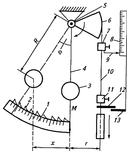
Рис. 3.17. Принципиальная схема разрывной машины с маятниковым силоизмерителем
