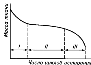
Рис. 4.48. Кривая изменения массы ткани при истирании
