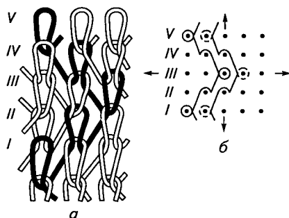
Рис. 4.11. Переплетение атлас:
