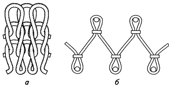
Рис. 4.7. Ластик 1+1:
