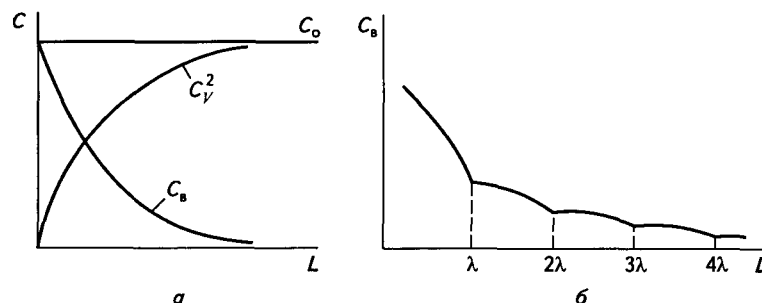
Рис. 5.8. Градиент неровноты: а — случайной; б — периодической
