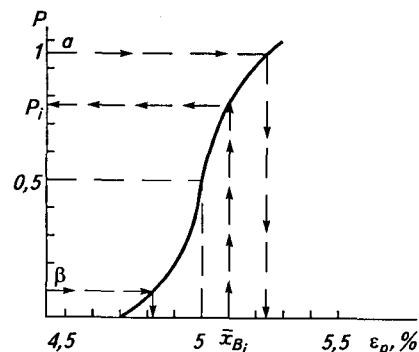
Рис. 5.5. Кривые вероятности приемки по удлинению при разрыве нити X_6
