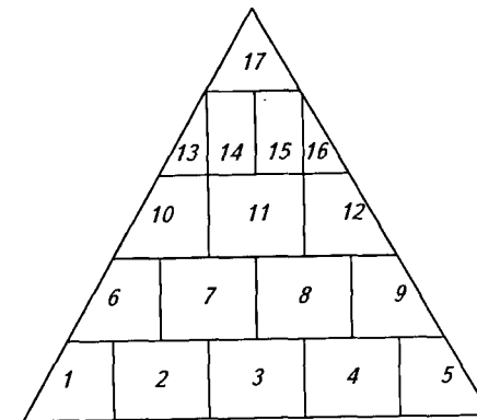
Рис. 5.12. Треугольник Файгенбаума:
