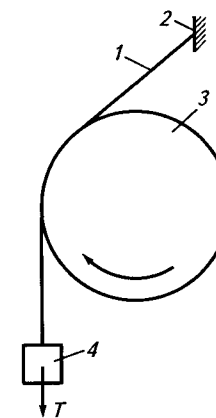
Рис. 2.14. Схема прибора для истирания волокон
