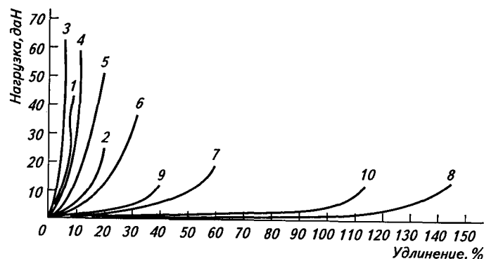
Рис. 4.19. Диаграммы «нагрузка — удлинение» (нечетными цифрами обозначены кривые удлинения материалов по основе или длине, четными — по утку или ширине): 1, 2 — хлопчатобумажная ткань; 3, 4 — льняное полотно; 5, 6 — хлопчатобумажная или шерстяная ткань; 7, 8 — трикотажное хлопчатобумажное (гладь) полотно; 9, 10 — нетканое хлопчатобумажное холстопршивное полотно
