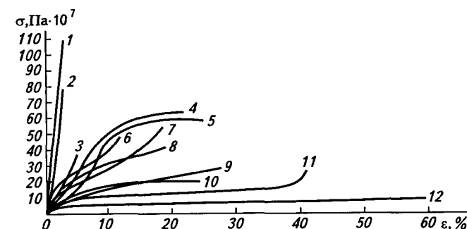
Рис. 3.15. Кривые растяжения волокон:
