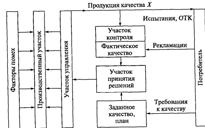
Рис. 5.10. Блок-схема УКП на стадии производства
