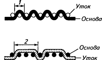
Рис. 4.1. Перекрытия нитей: 1 — основное; 2 — уточное
