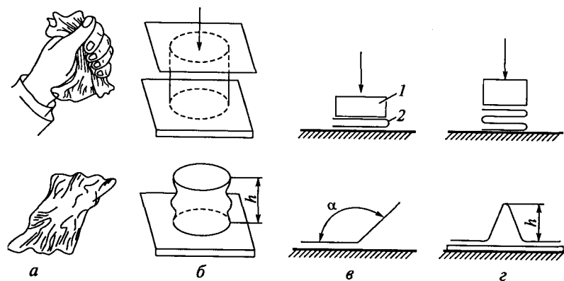
Рис. 4.30. Определение степени несминаемости тканей
