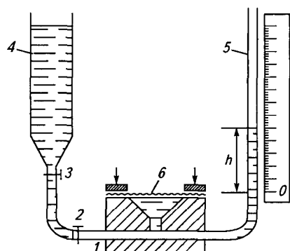
Рис. 4.43. Определение водоупорности методом «кошеля»
