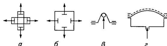
Рис. 4.22. Методы двухосного (а, б) и многоосного (в, г) растяжения материалов
