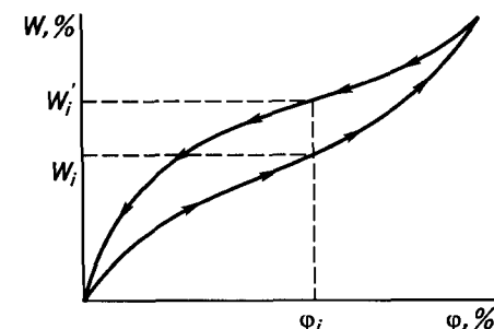
Рис. 2.15. Изотермы сорбции и десорбции влаги
