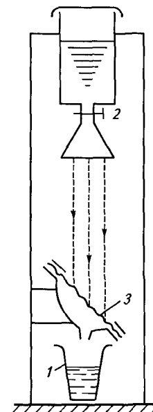
Рис. 4.41. Схема дождевальной установки
