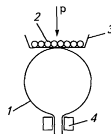
Рис. 4.27. Определение жесткости тканей при изгибе методом кольца
