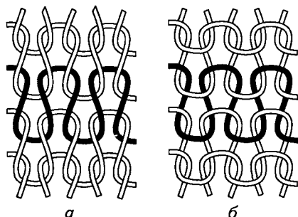
Рис. 4.6. Гладь. Стороны:
