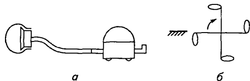
Рис. 4.40. Определение пылепроницаемости
