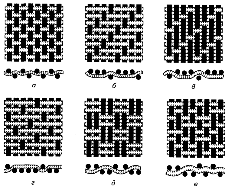
Рис. 4.3. Виды переплетений:
