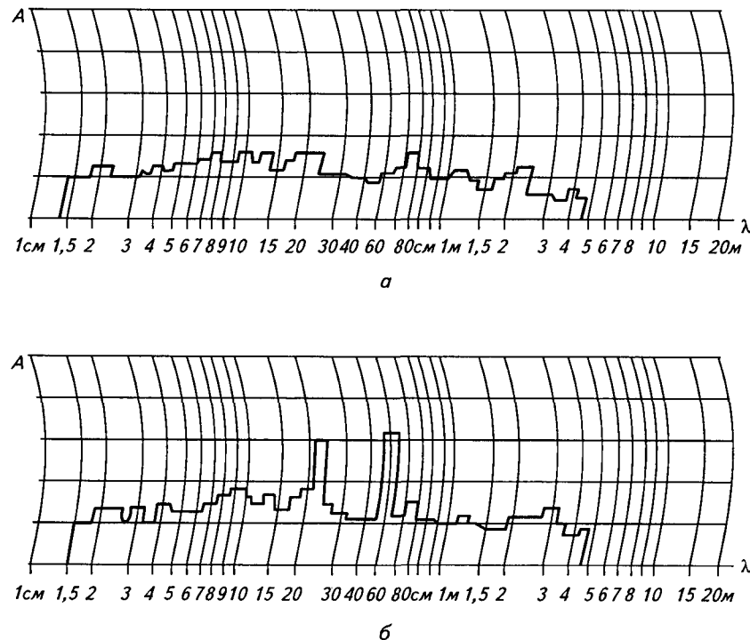
Рис. 3.13. Спектрограммы:
