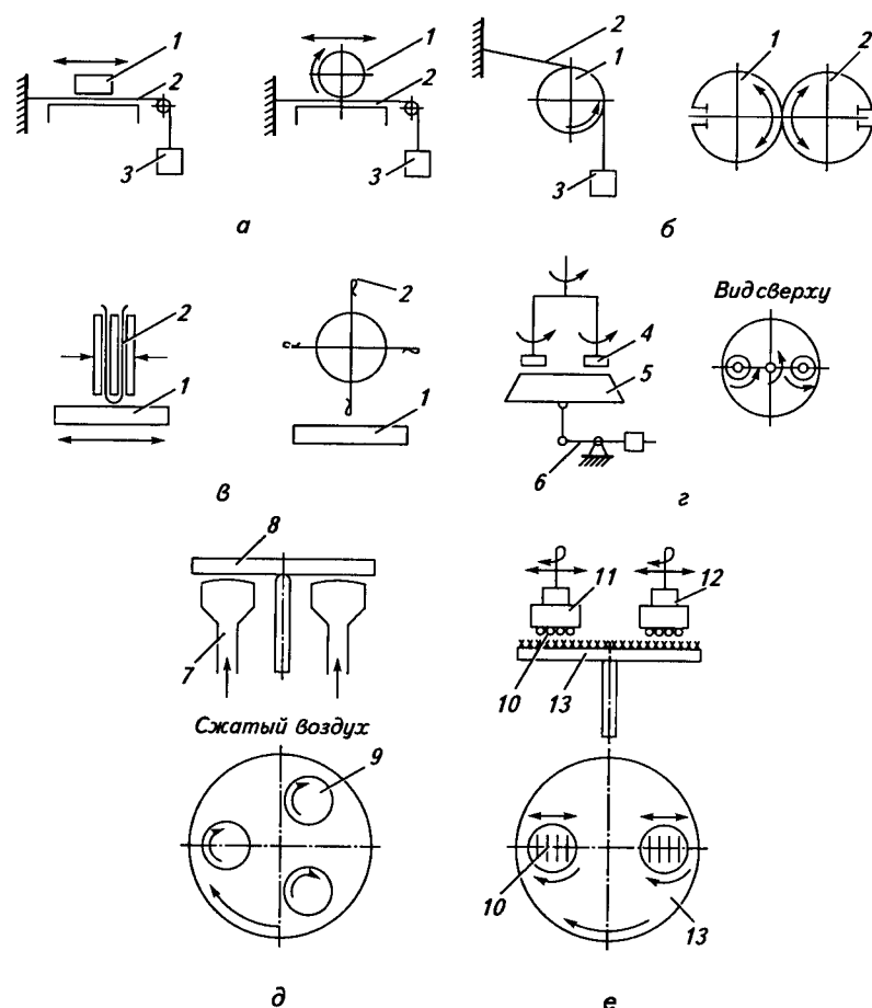
Рис. 4.49. Определение стойкости тканей к истиранию различными методами
