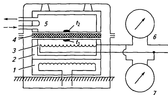
Рис. 4.44. Схема стандартного прибора для определения теплозащитных свойств изделий методом стационарного режима
