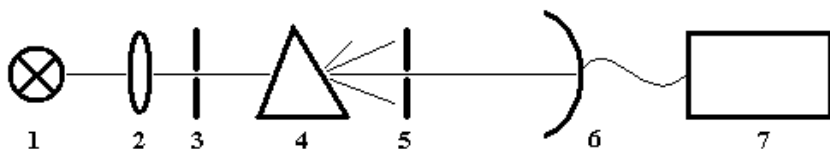
Рис. 6.11. Схема спектрометра с призмennым монохроматором: 1 – источник света; 2 – фокусирующая оптика; 3 – входная щель; 4 – призма; 5 – выходная щель; 6 – приемник (фотоэлемент); 7 – регистрирующее устройство (микроамперметр и т. п.)
