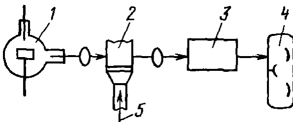
Рис. 6.17. Схема ААС-спектрометра с пламенным атолизатором
