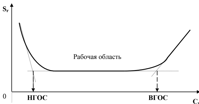
Рис. 2.2. Связь воспроизводимости анализа с концентрацией определяемого компонента
