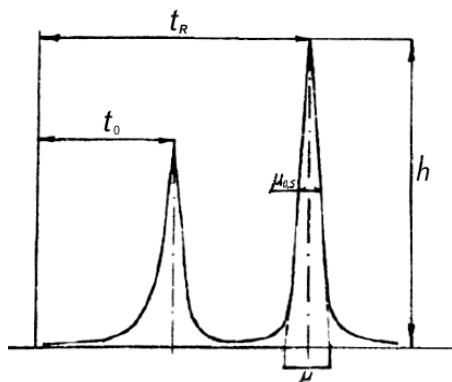
Рис. 7.10. Параметры хроматографического пика
