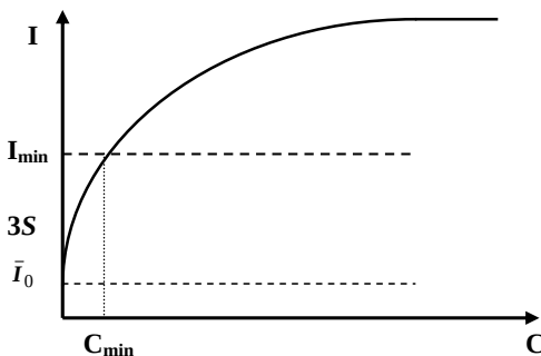
Рис. 5.3. Статистическая оценка предела обнаружения по градуировочному графику
