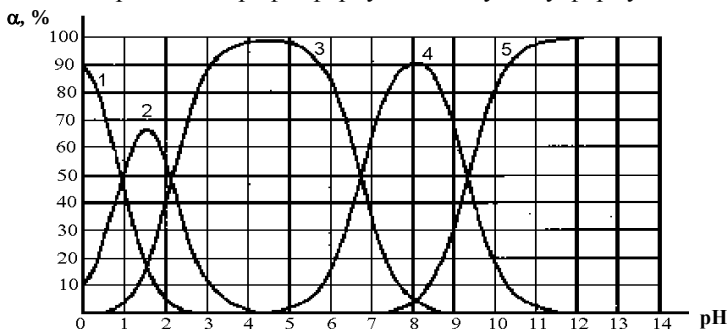
Рис. 3.6. Состояние пиродифосфорной кислоты в водном растворе: 1 – \text{H}_4\text{R} ; 2 – \text{H}_3\text{R}^- ; 3 – \text{H}_2\text{R}^{2-} ; 4 – \text{HR}^{3-} ; 5 – \text{R}^{4-}
