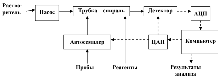
Рис. 5.4. Схема автоматического анализатора для проточно-инжекционного анализа
