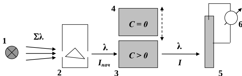
Рис. 6.20. Принципиальная схема однолучевого спектрофотометра: 1 – источник света; 2 – призменный монохроматор; 3 – кювета с исследуемым раствором; 4 – кювета с раствором сравнения; 5 – приемник света (фотоэлемент); 6 – микроамперметр
