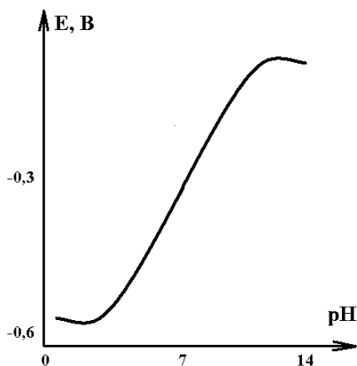
Рис. 6.3. Зависимость потенциала стеклянного электрода от pH раствора (при 25 °С)
