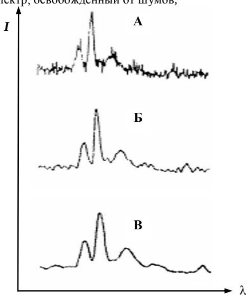
Рис. 9.2. Спектры поглощения в ИК-области, полученные при однократной регистрации без сглаживания (А) и с применением сглаживающего фильтра (В), а также усредненные по результатам 10-кратной регистрации без фильтра (Б)
