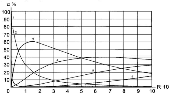
Рис. 3.7. Распределительная диаграмма для процесса образования роданидных комплексов железа(III) 1 – M ; 2 – MR_1 ; 3 – MR_2 ; 4 – MR_3 ; 5 – MR_4 ; 6 – MR_5 ; 7 – MR_6
