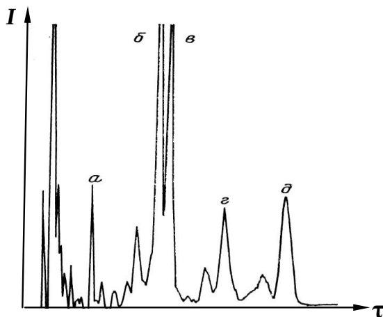
Рис. 7.4. Участок хроматограммы экстракта из мышечной ткани.
