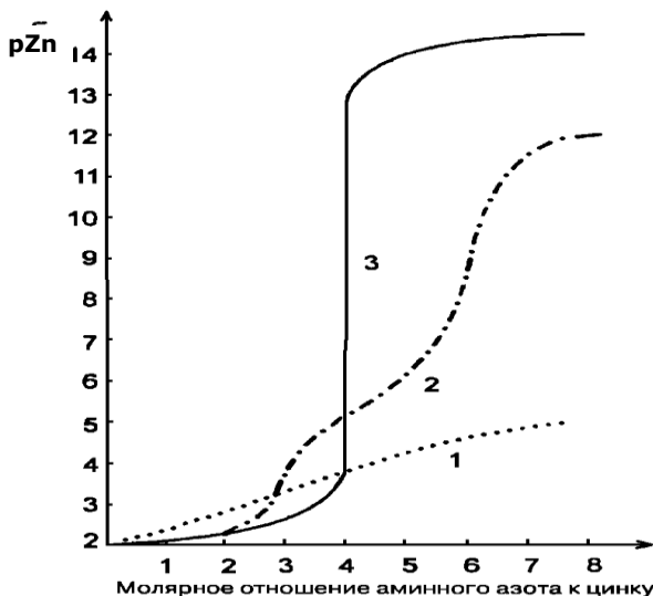
Рис. 4.12. Кривые титрования катионов цинка аммиаком (1), этилендиамином (2) и триэтилентетрамином (3)
