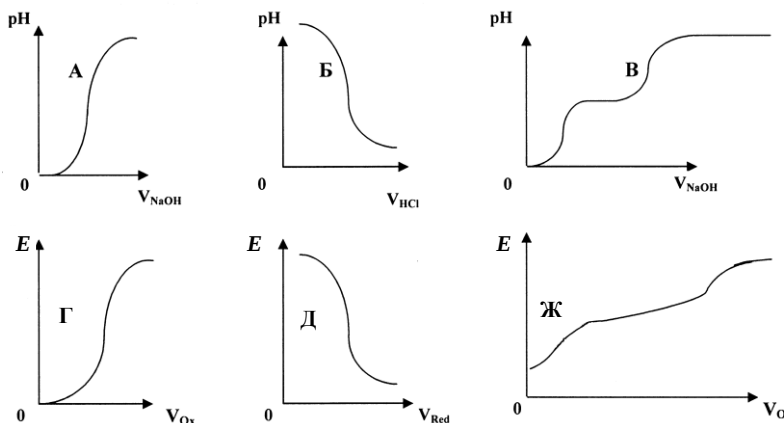
Рис. 4.7. Логарифмические кривые для разных случаев кислотно-основного (вверху) и окислительно-восстановительного (внизу) титрования:
